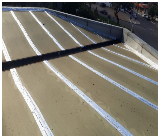
Figura 6: Pontos da chapa de policarbonato apresentando perfurações e tonalidade amarelada na cobertura da recepção principal de entrada, ocasionando infiltrações.
